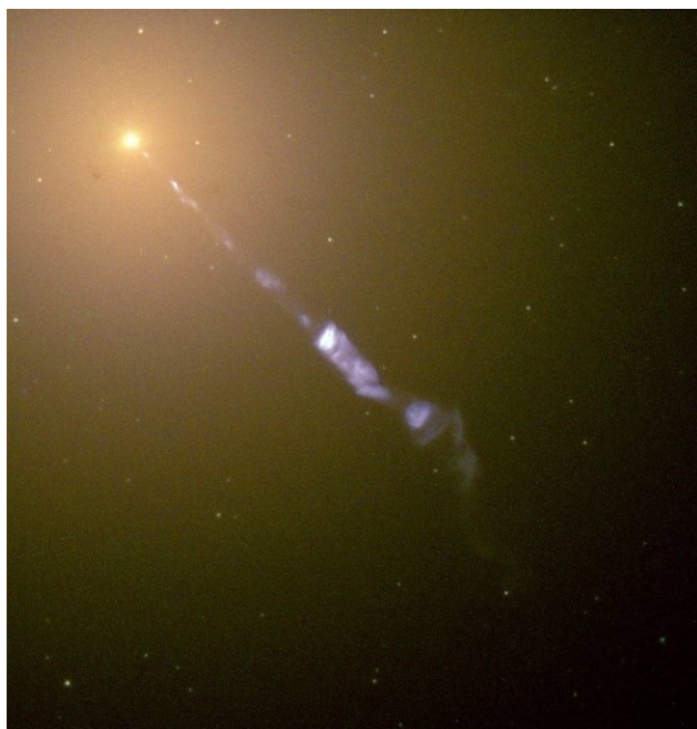
Synchrotron - quasars
